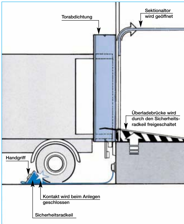
Bild 8-2: Beispiel einer Überladebrücke mit Sicherung durch Radkeil
