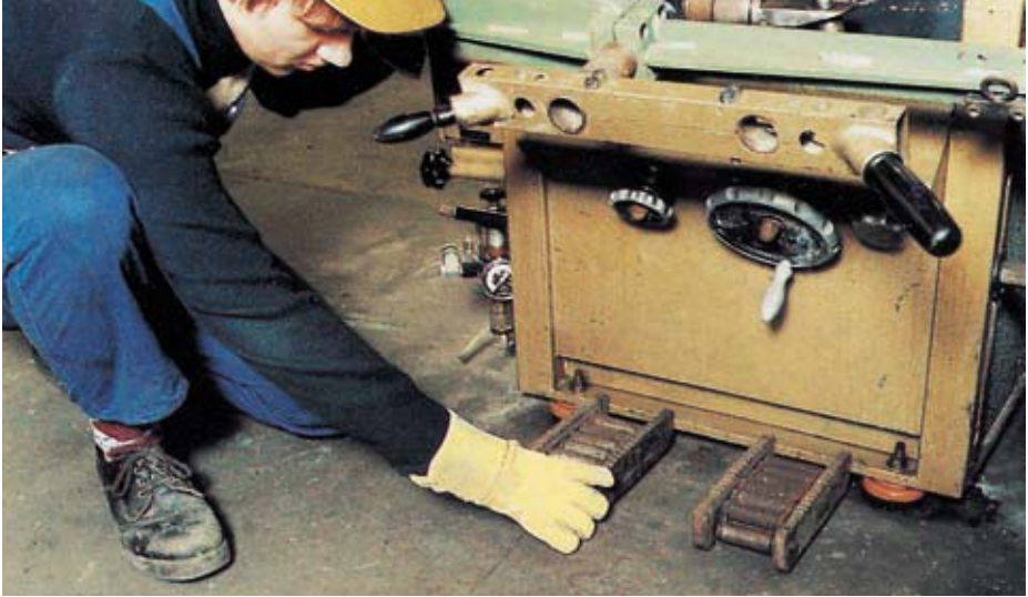
Bild 4-6: Transportfahrwerke
