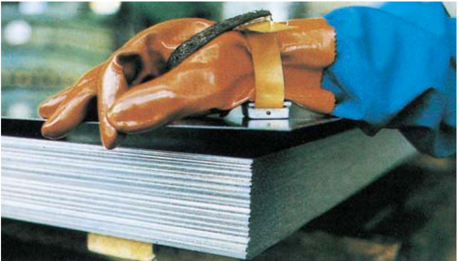
Bild 17-4: Kunststoffbeschichteter Schutzhandschuh und Handmagnet im Einsatz
